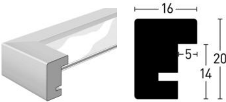
Max. Einlegehöhe 2,3 mm | Max. insertion height 2,3 mm
