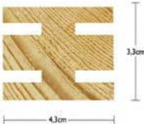
Mittelstrebe | Centre strut
