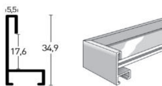
Profil 34 Natura | Profile 34 Natura
