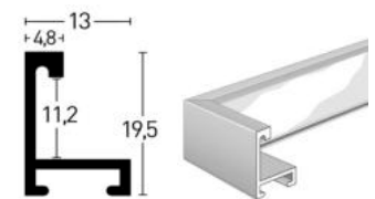
Profil 273 | Profile 273 Natura
