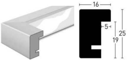
Max. Einlegehöhe 7 mm | Max. insertion height 7 mm
