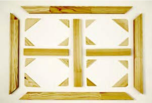
Zusammenbau eines 19 mm Rahmens mit Stützkreuz Assembling of a 19 mm frame with supporting cross struts
